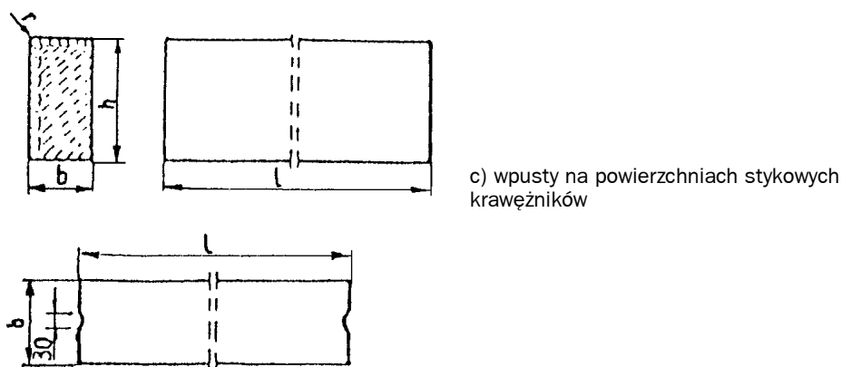
Rys. 1. Wymiarowanie krawężników
